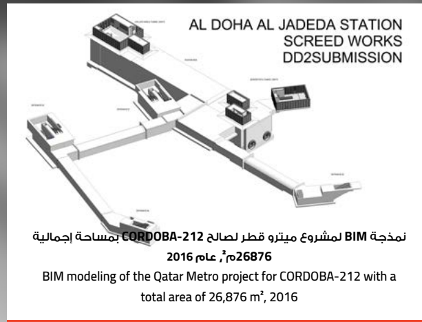
مشروع مترو قطر.. الخط الذهبي Qatar Metro Project..Golden Line
